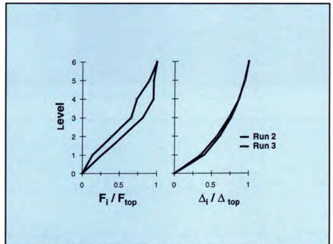
(d) Lateral force distributions and deflected shapes
