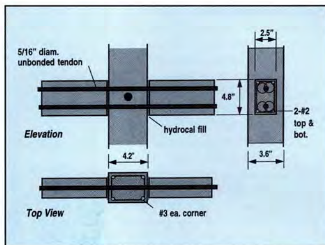
(d) Detail of post-tensioned connection
