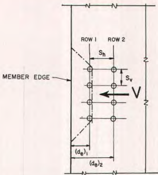
Fig. 18. Stud group under shear.
