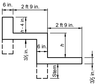
Double riser
